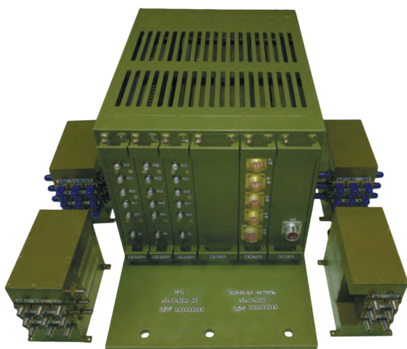
3-канальный преобразователь частоты диапазона 0,1 - 18,0 ГГц, серии Радиотехника-1.
