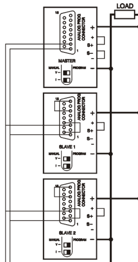
Параллельное подключение
