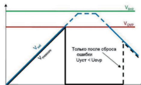
Функционирование в режиме OVP
