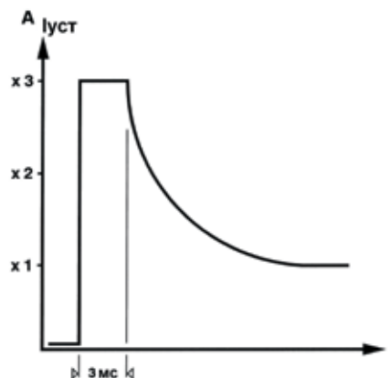
Трехкратный импульсный выходной ток (с опцией КЗ нагрузки ТОЕ 7610/103)
